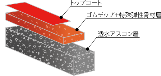
■パーフェクトジョギングAF-J断面図
