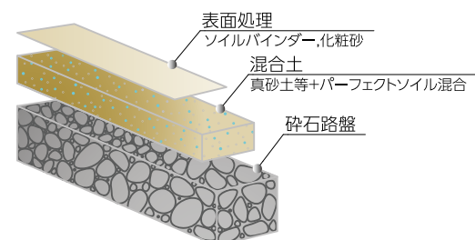
■ソイルサンドクレイ断面図
