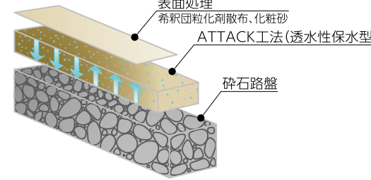
■ATTAC工法断面図
