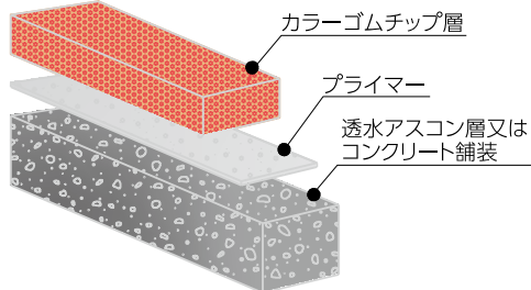
■パーフェクトプロムナード断面図
