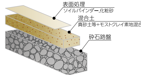
■モストクレイ断面図
